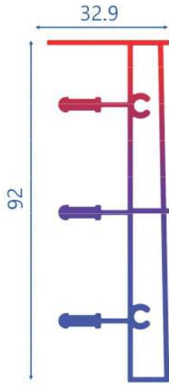
T.2352 1.377 KG/MT 3 KANALLI ALT KASA
