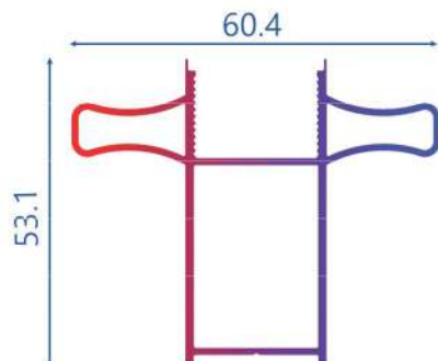
T.2358 - 0.852 KG/MT ÇİFT TARAFLI TUTAMAK
