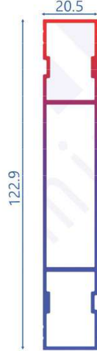
T.2363 1.272 KG/MT 4 KANALLI YAN KASA
