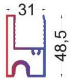
T.2490 - 0,898 KG/MT
