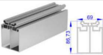
ORTA TAŞIYICI PROFİLİ MIDDLE BEAM PROFILE STOK KODU: SG-1020 2,60 KG/ 86,73x69,8x2mm
