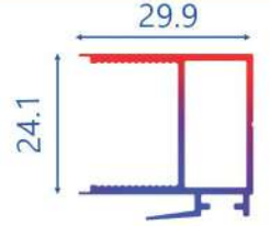
T.2356 - 0.406 KG/MT ÇEKME BAZA PROFİLİ
