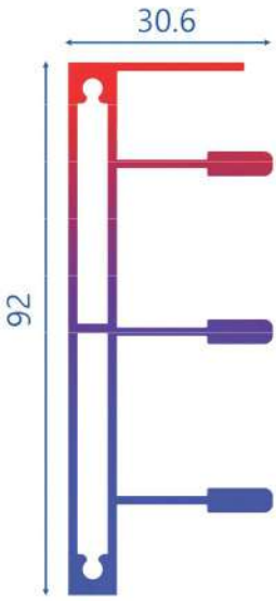
T.2351 1.642 KG/MT 3 KANALLI ÜST KASA
