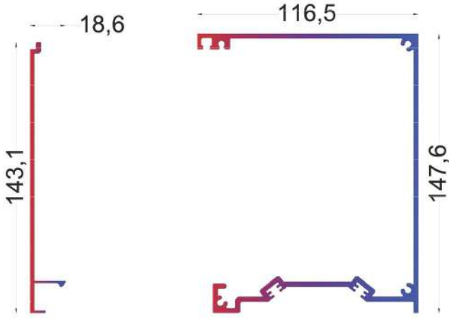
T.2402 - 0,915 KG/MT
