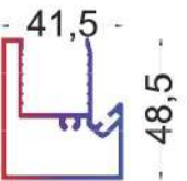
T.2492 - 0,871 KG/MT
