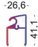
T.2467 - 0,673 KG/MT
