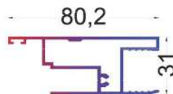
T.2493 - 0,999 KG/MT
