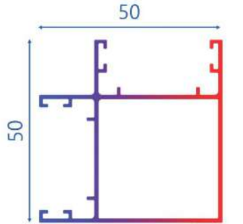
T.2360 - 0.748 KG/MT KOŞE DÖNÜŞ PROFİLİ
