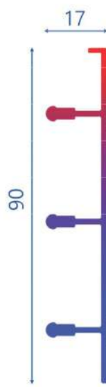
T.2365 0.807 KG/MT 3 KANALLI EŞİKSİZ ALT KASA
