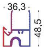
T.2491 - 0,917 KG/MT
