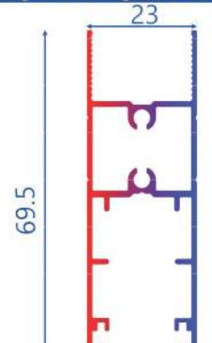
T.2360 - 0.748 KG/MT KOŞE DÖNÜŞ PROFİLİ
