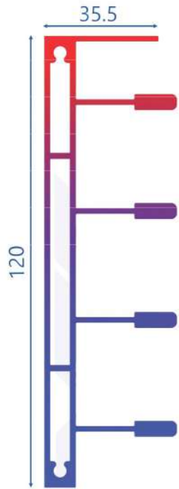
T.2361 2.108 KG/MT 4 KANALLI ÜST KASA
