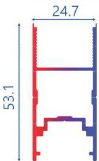
T.2367 - 0.674 KG/MT SÜRME İSPANYOLET PROFİLİ
