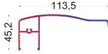
T.2450 - 1,132 KG/MT
