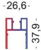
T.2457 - 0,647 KG/MT
